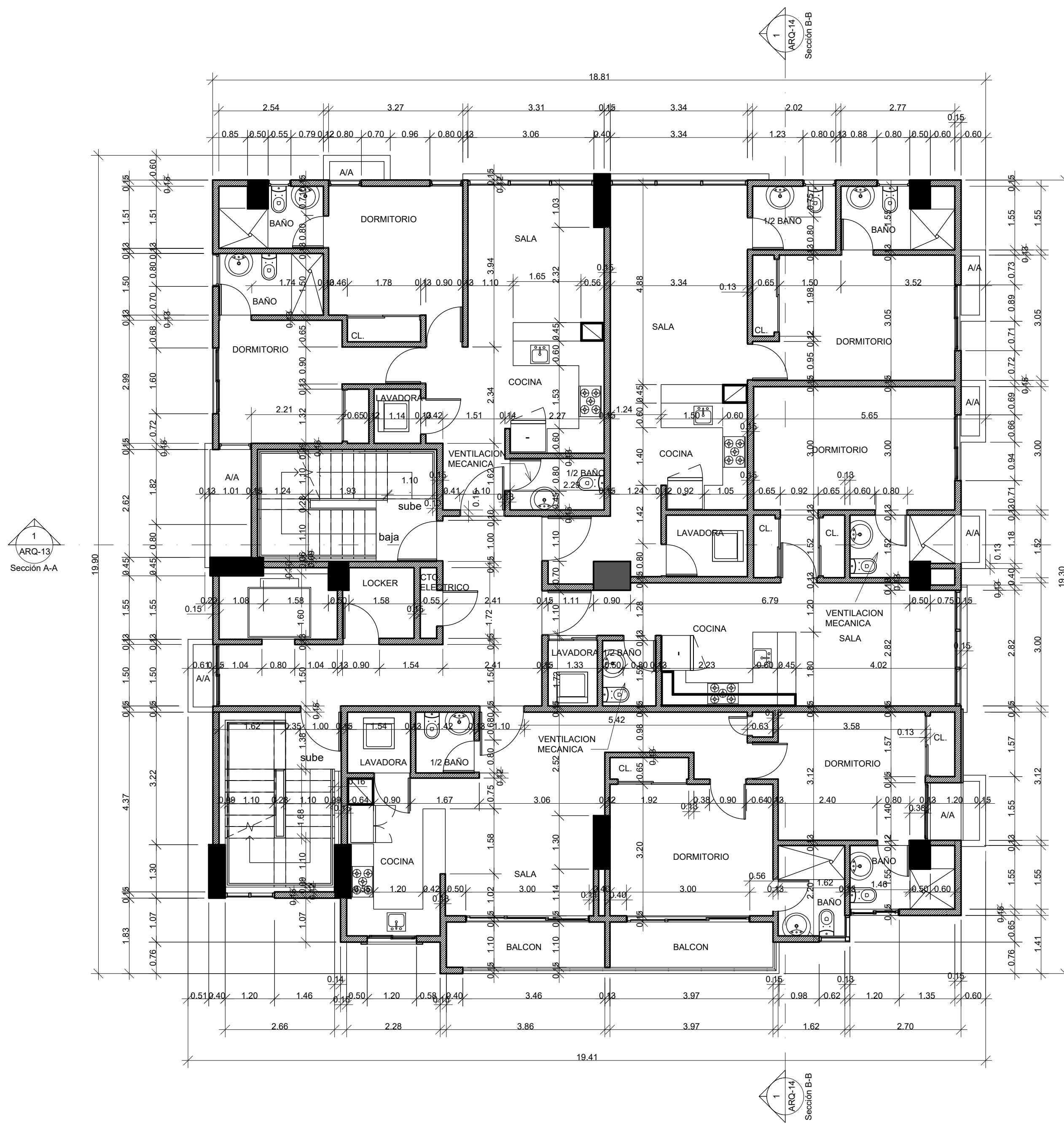
1 PLANTA ARQ. DIMENSIONADA 3er. @ 10mo. NIVEL 1 : 75
